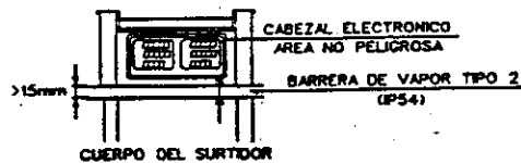
DETALLE "C"
