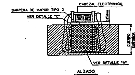
ALZADO
